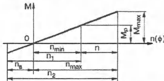
Рис. 2. Теоретична діаграма роботи плоскої спіральної пружини
