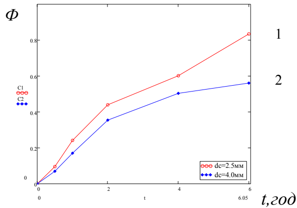
Рис. 5. \Phi = f(t) в апараті з мішалкою при T = 40^\circ \text{C} (1- d_c=2,5\text{мм} ; 2- d_c=4,0 )
