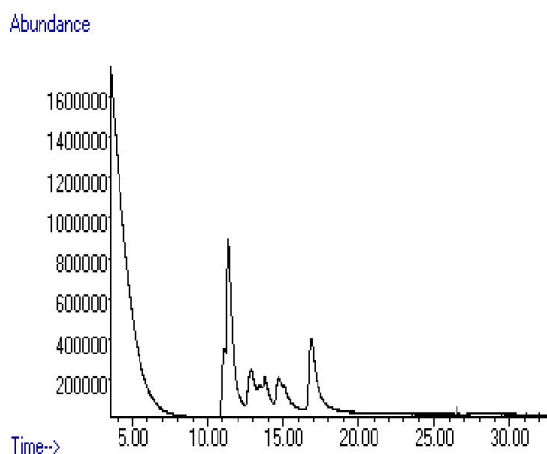
Рис. 13. Хроматограма CO 2 -екстракту біомаси G. imbricatus
