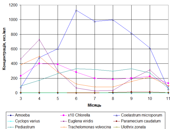
Рис. 7. Графіки концентрації мікропланктону в воді оз. Басів Кут, отримані в результаті вимірювань розробленим пристроєм
